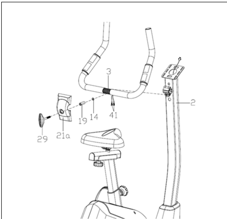
Рисунок 6 – Установка руля
