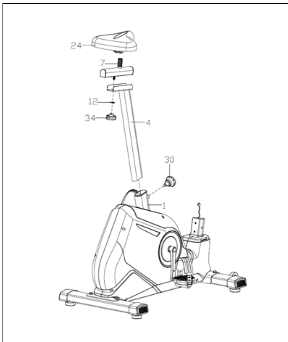
Рисунок 4 – Установка сиденья
