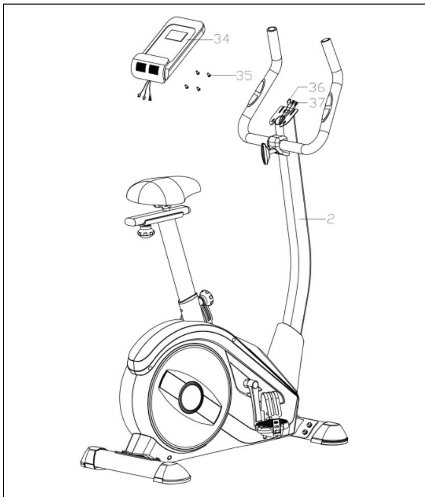
Рисунок 7 – Установка консоли
