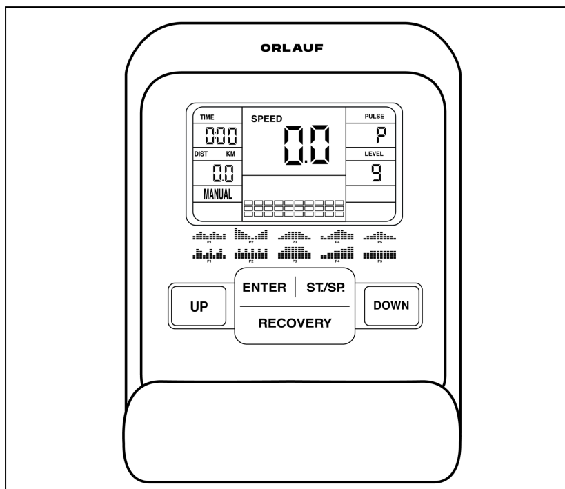
Рисунок 8 – Консоль велотренажера
