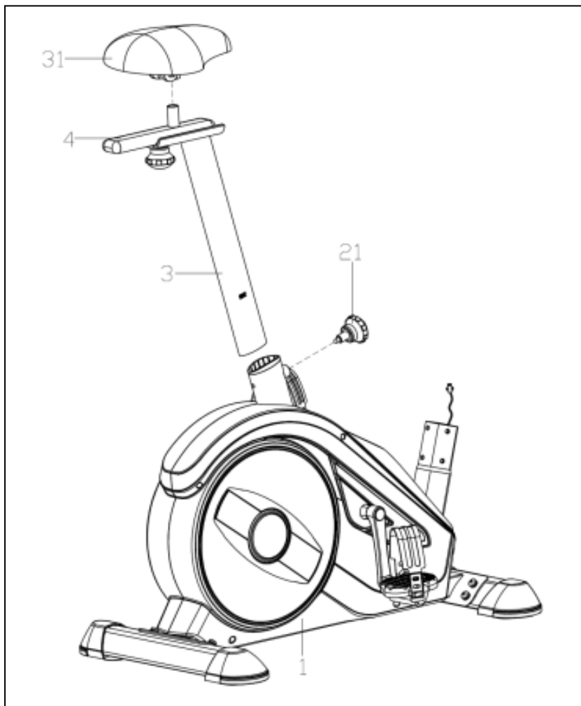
Рисунок 4 – Установка сиденья
