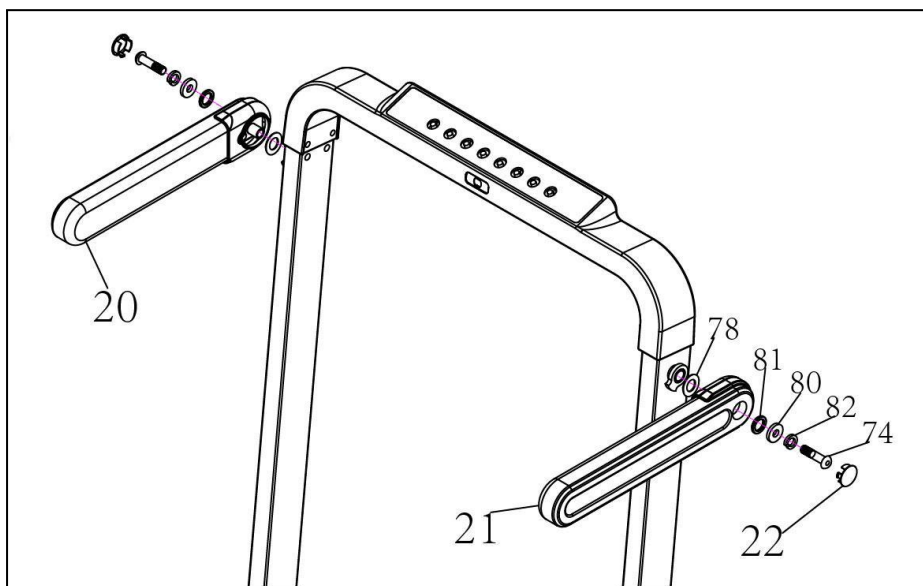
Рисунок 4 — Фиксация поручней
